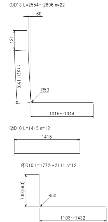
鉄筋加工図
