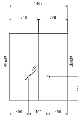
正面構造図
