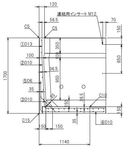
断面配筋図
