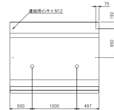
背面構造図
