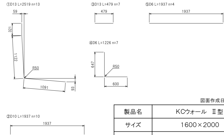
鉄筋加工図
