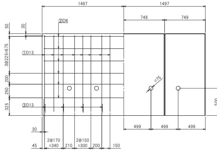
たて壁配筋図
