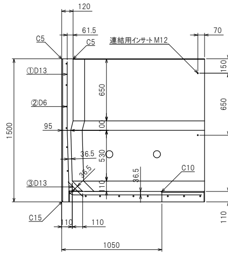
断面配筋図
