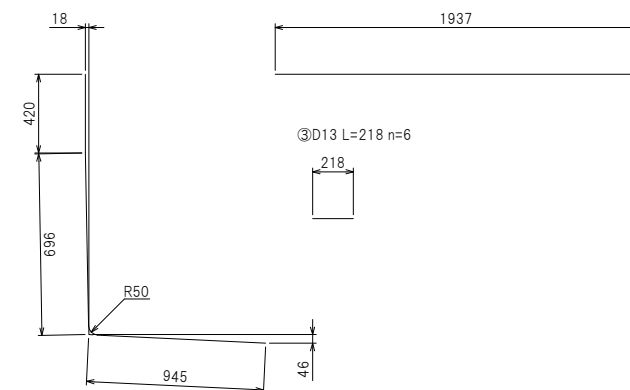
鉄筋加工図
