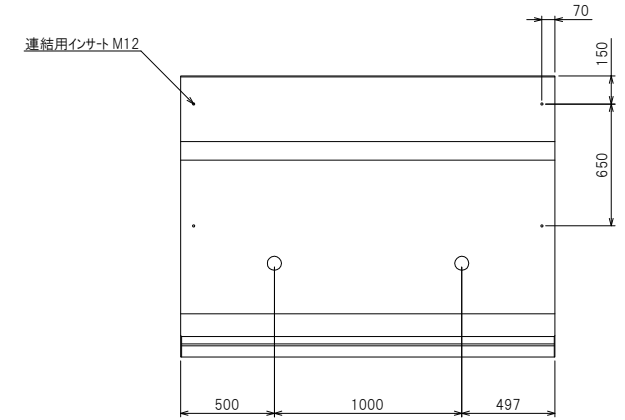
背面構造図
