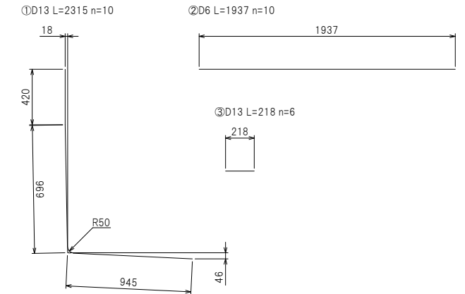
鉄筋加工図
