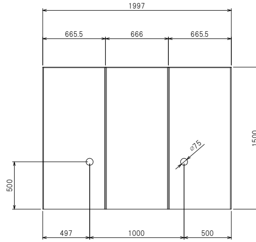
正面配筋図
