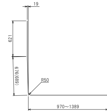
鉄筋加工図
