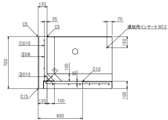
断面配筋図
