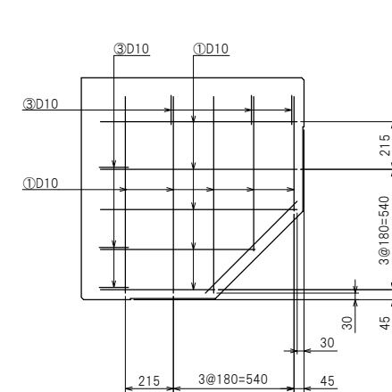
底板配筋図
