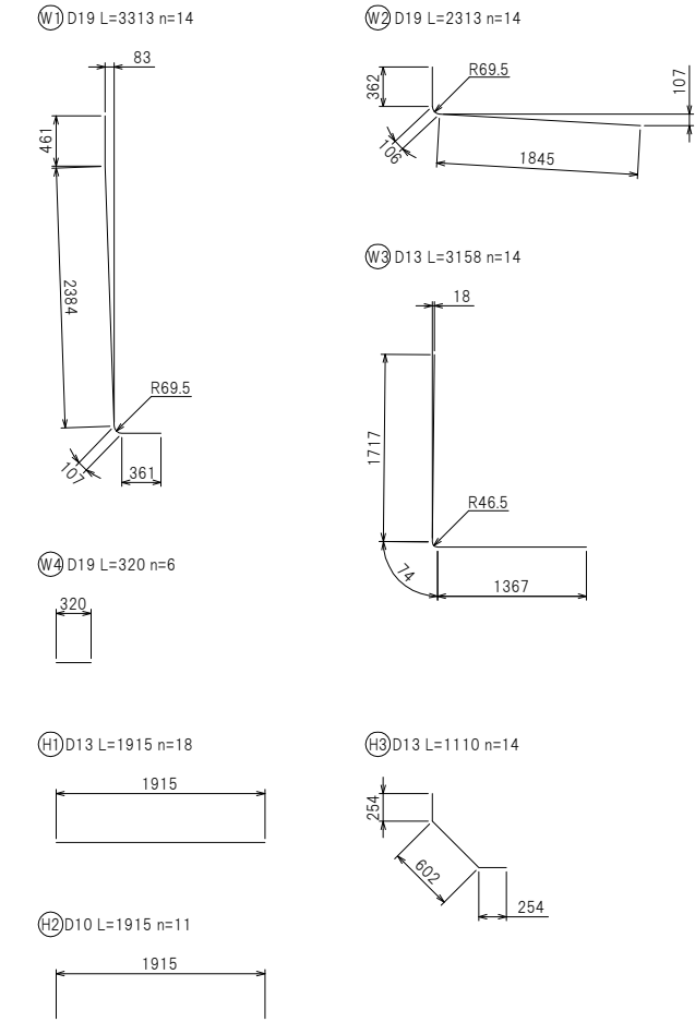
鉄筋加工図
