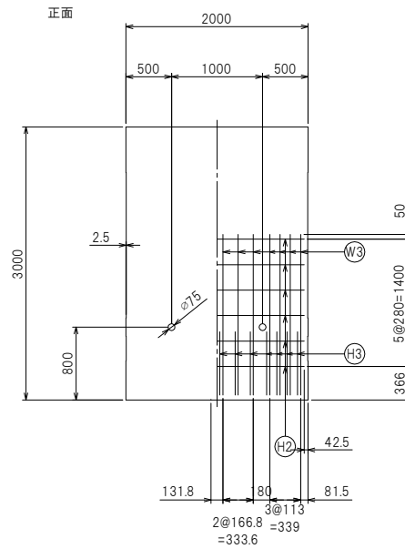
たて壁配筋図
