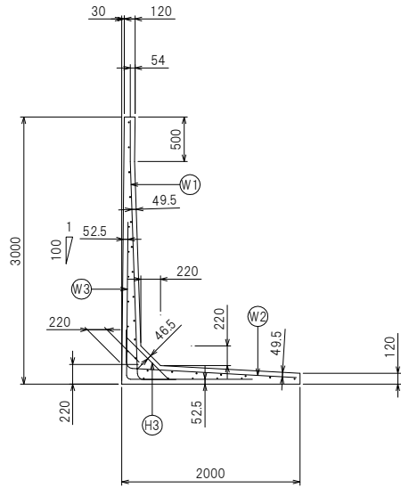
断面配筋図
