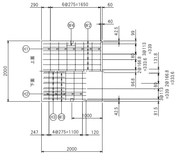
底板配筋図
