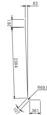
鉄筋加工図
