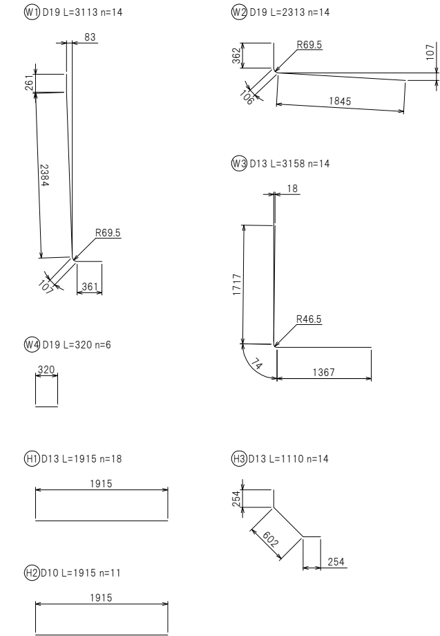
鉄筋加工図
