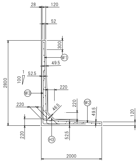
断面配筋図
