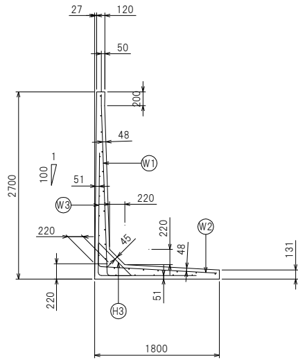
断面配筋図
