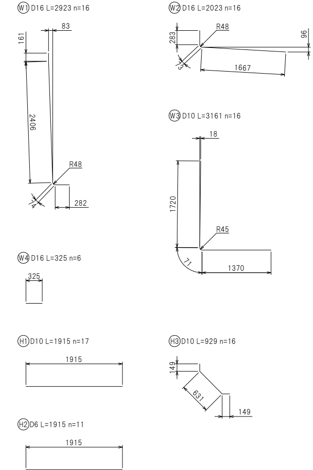
鉄筋加工図
