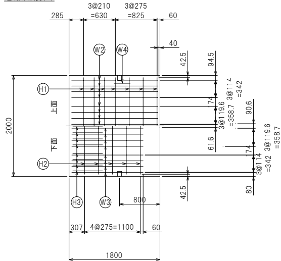
底板配筋図
