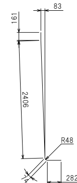
鉄筋加工図
