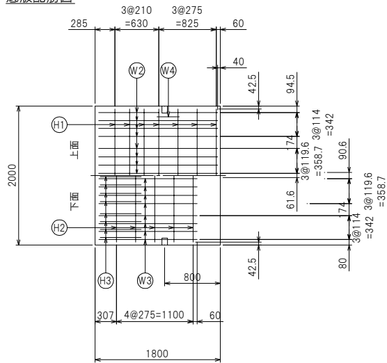
底板配筋図
