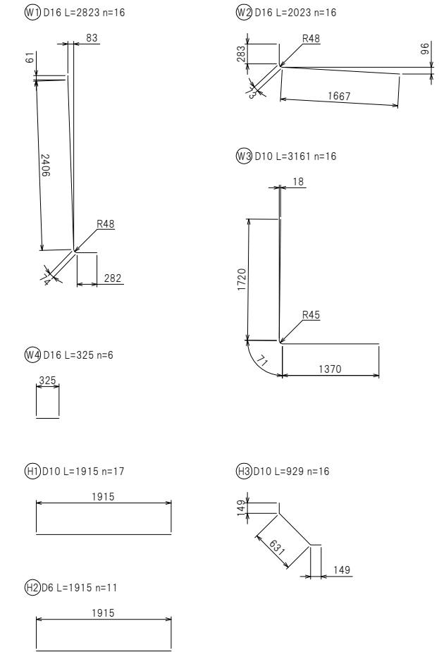
鉄筋加工図
