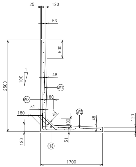
断面配筋図
