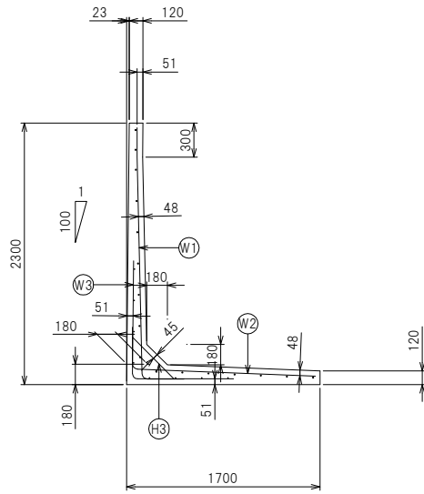
断面配筋図
