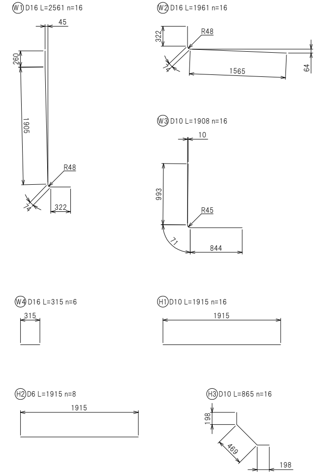
鉄筋加工図
