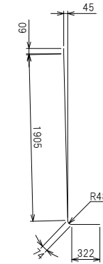
鉄筋加工図
