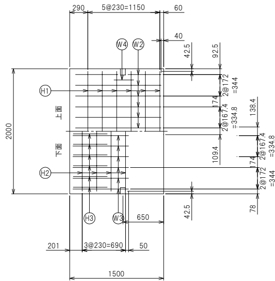
底板配筋図
