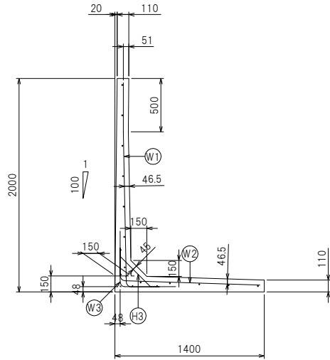
断面配筋図
