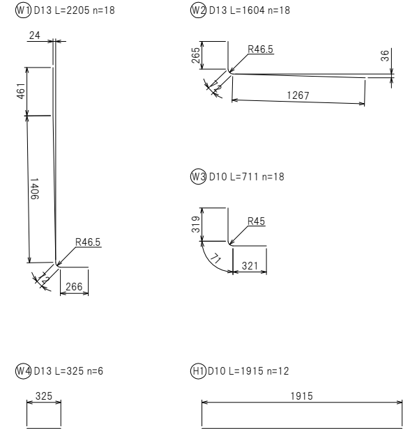
鉄筋加工図
