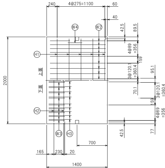
底板配筋図
