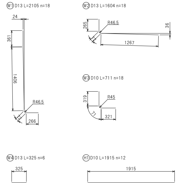
鉄筋加工図
