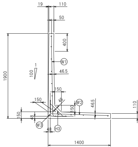
断面配筋図
