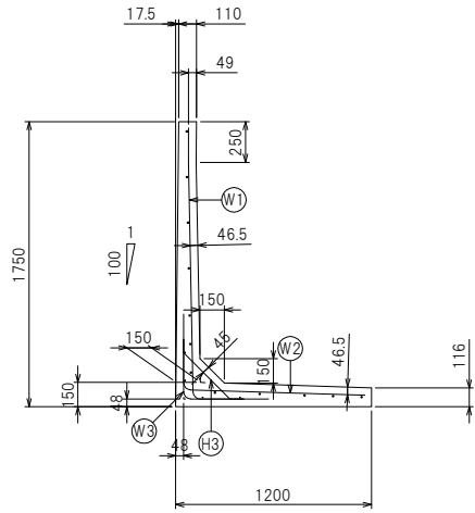
断面配筋図
