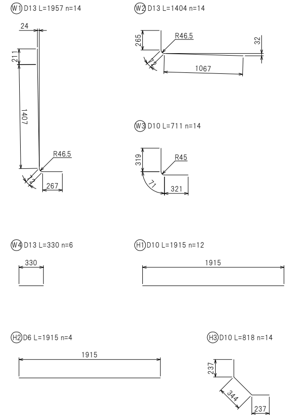
鉄筋加工図
