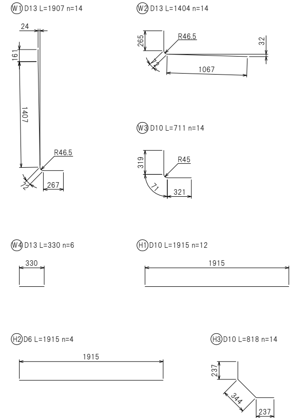
鉄筋加工図
