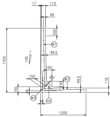
断面配筋図
