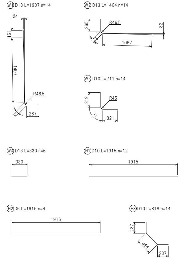
鉄筋加工図
