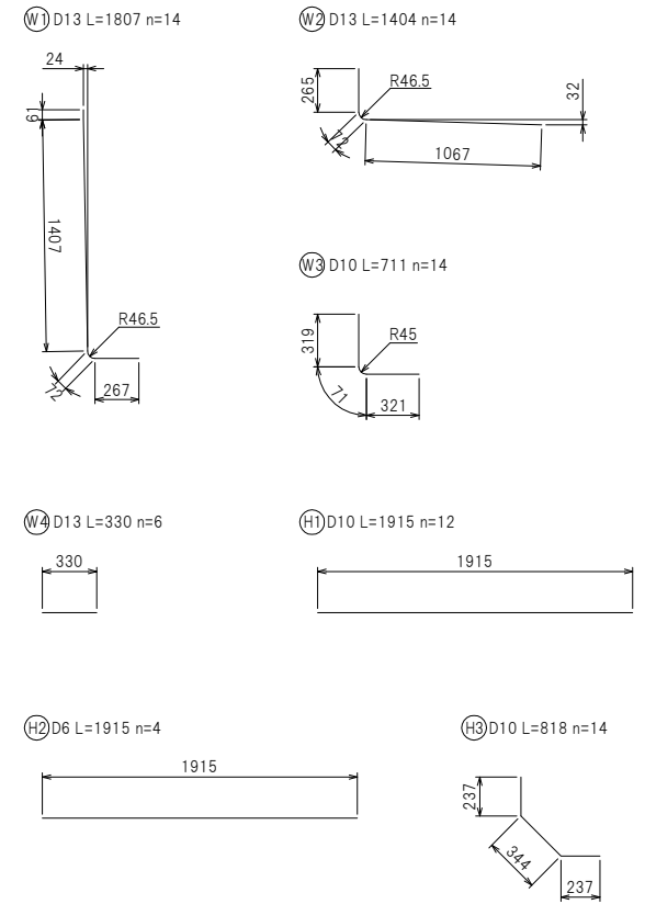
鉄筋加工図
