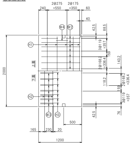
底板配筋図
