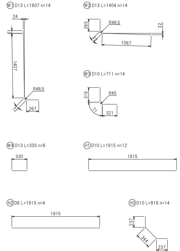
鉄筋加工図
