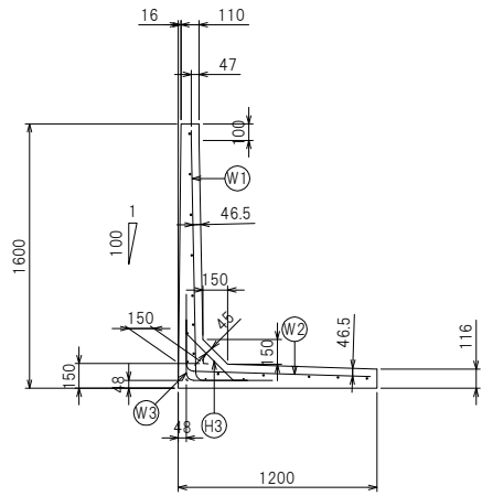
断面配筋図
