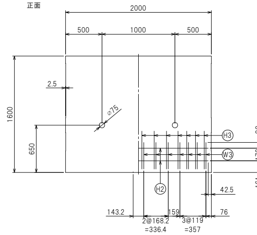
たて壁配筋図
