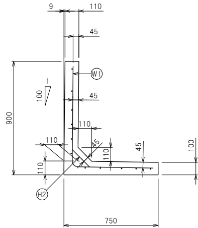
断面配筋図
