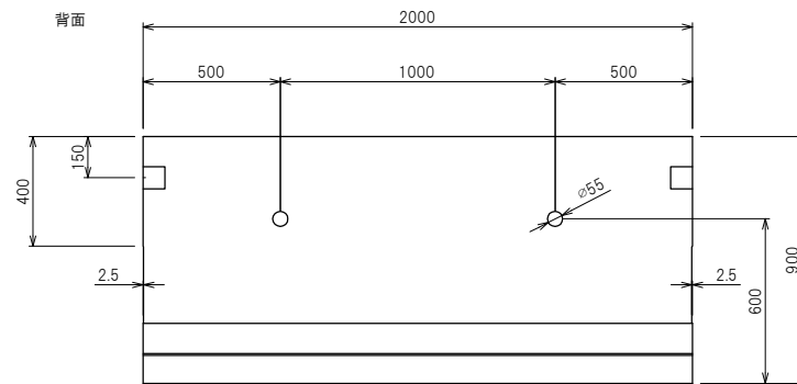
たて壁構造図
