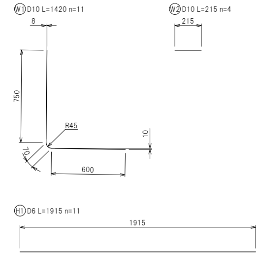
鉄筋加工図
