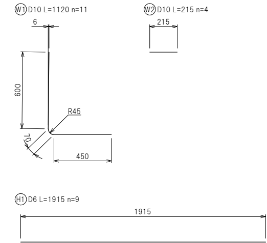
鉄筋加工図
