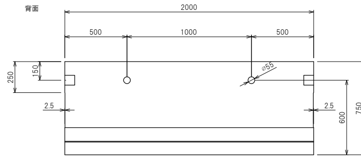
たて壁構造図
