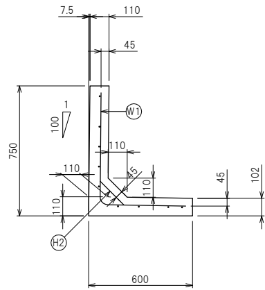
断面配筋図
