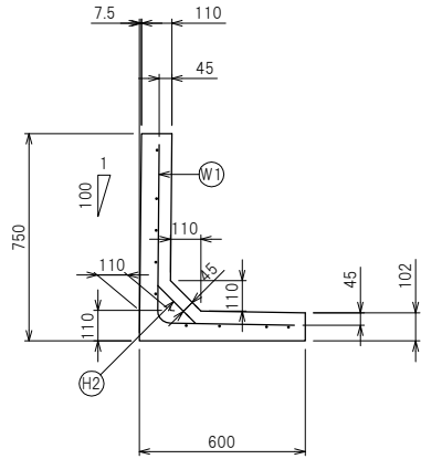
断面配筋図
